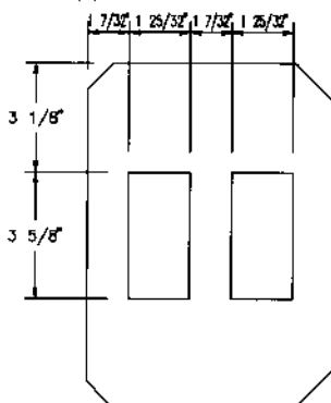
ETRB-82 (2) 1/8" DIN OPENINGS
